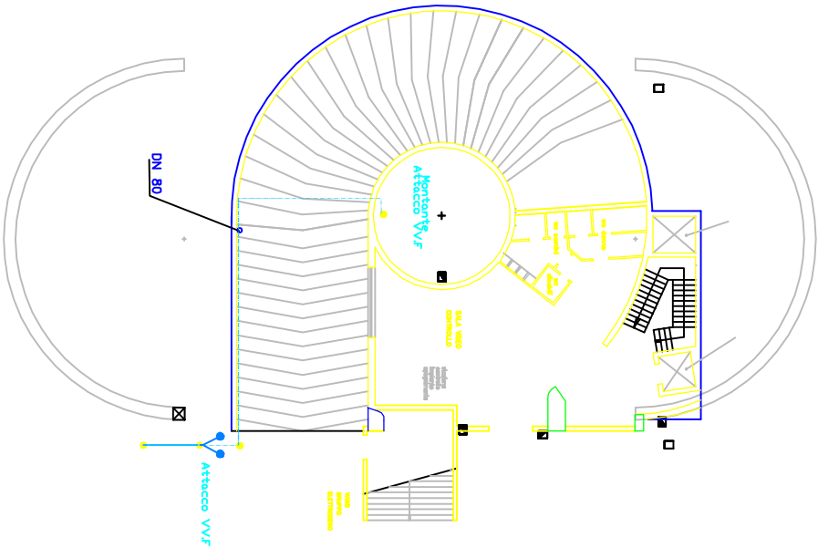
PIANTA PIANO SERVIZI PLANIMETRIA IMPIANTO SPRINKLER
