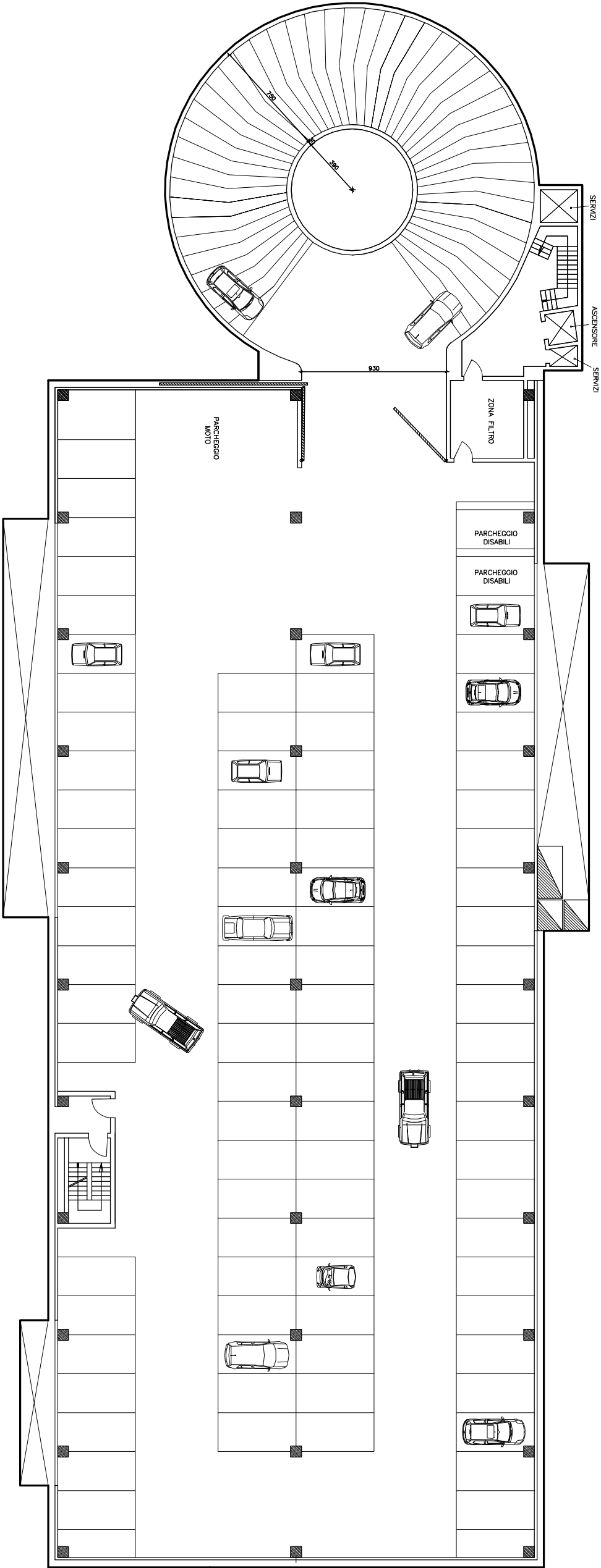
PIANTA SECONDO INTERRATO 1:100
