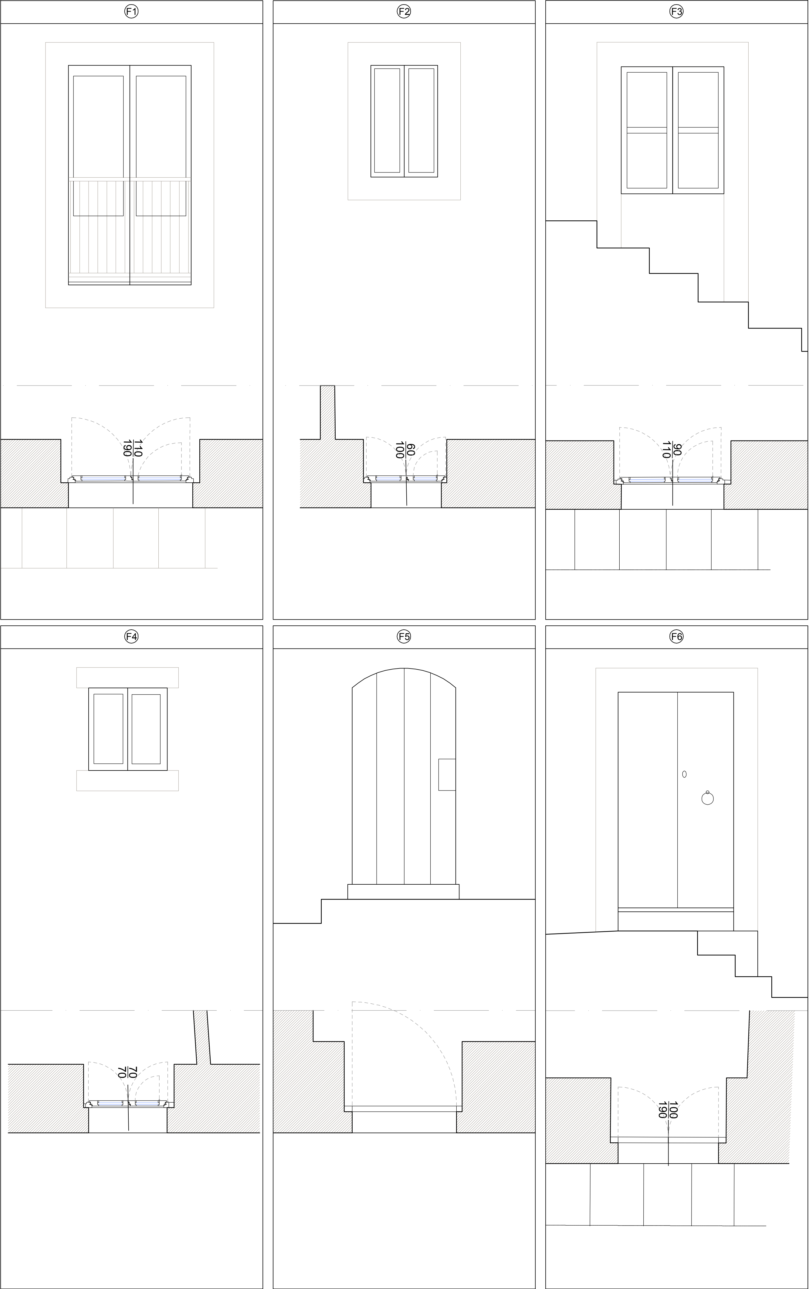
ABACO INFISSI scala 1:20
