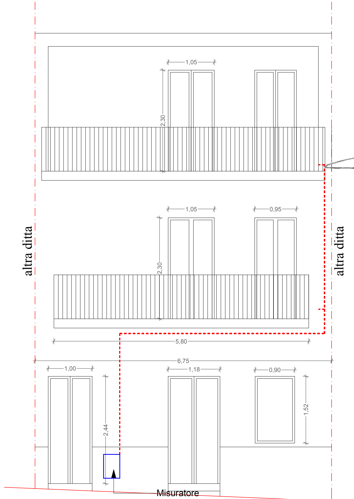
Prospetto su via Francesco Crispi
