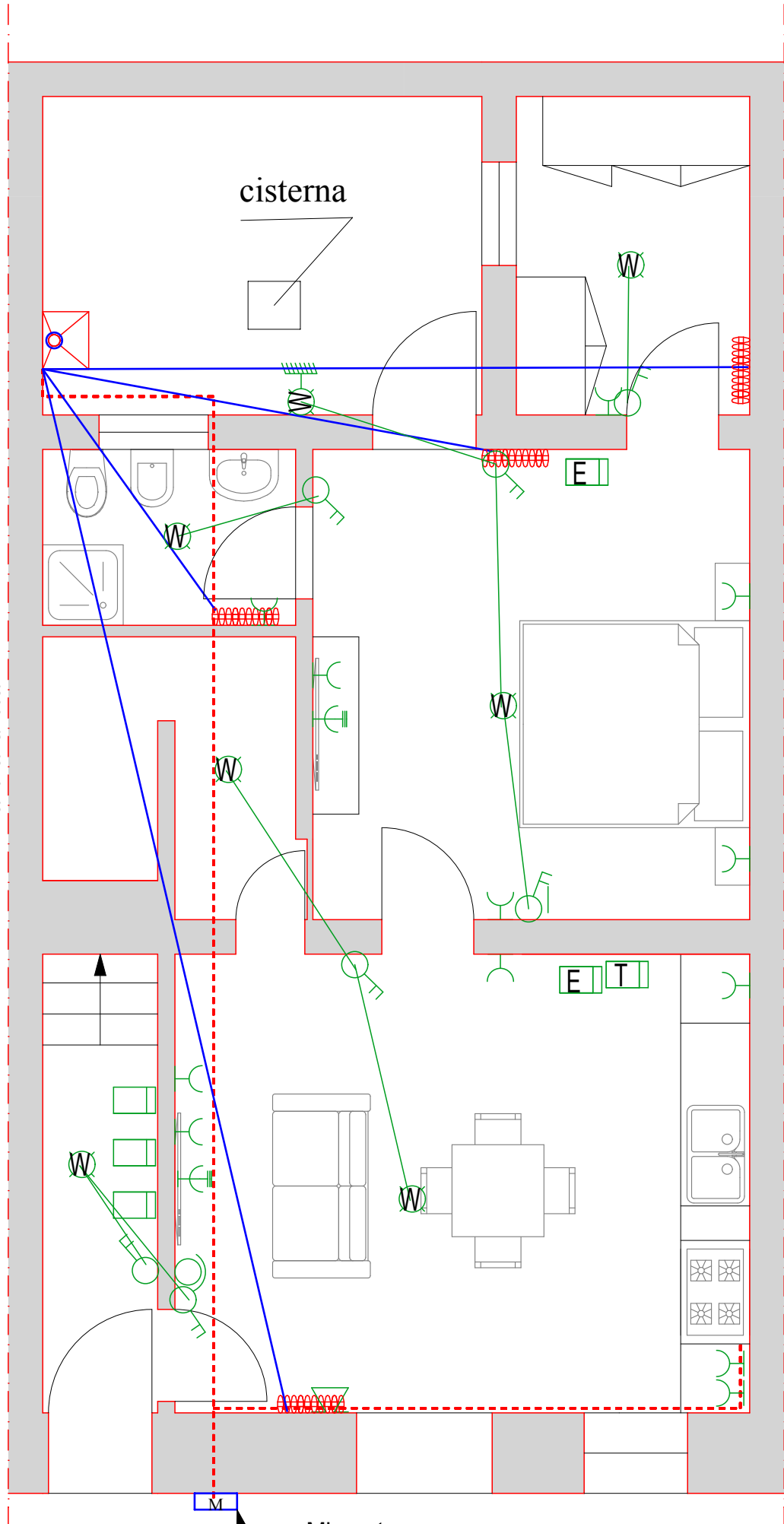
Impianto metano Piano Terra
