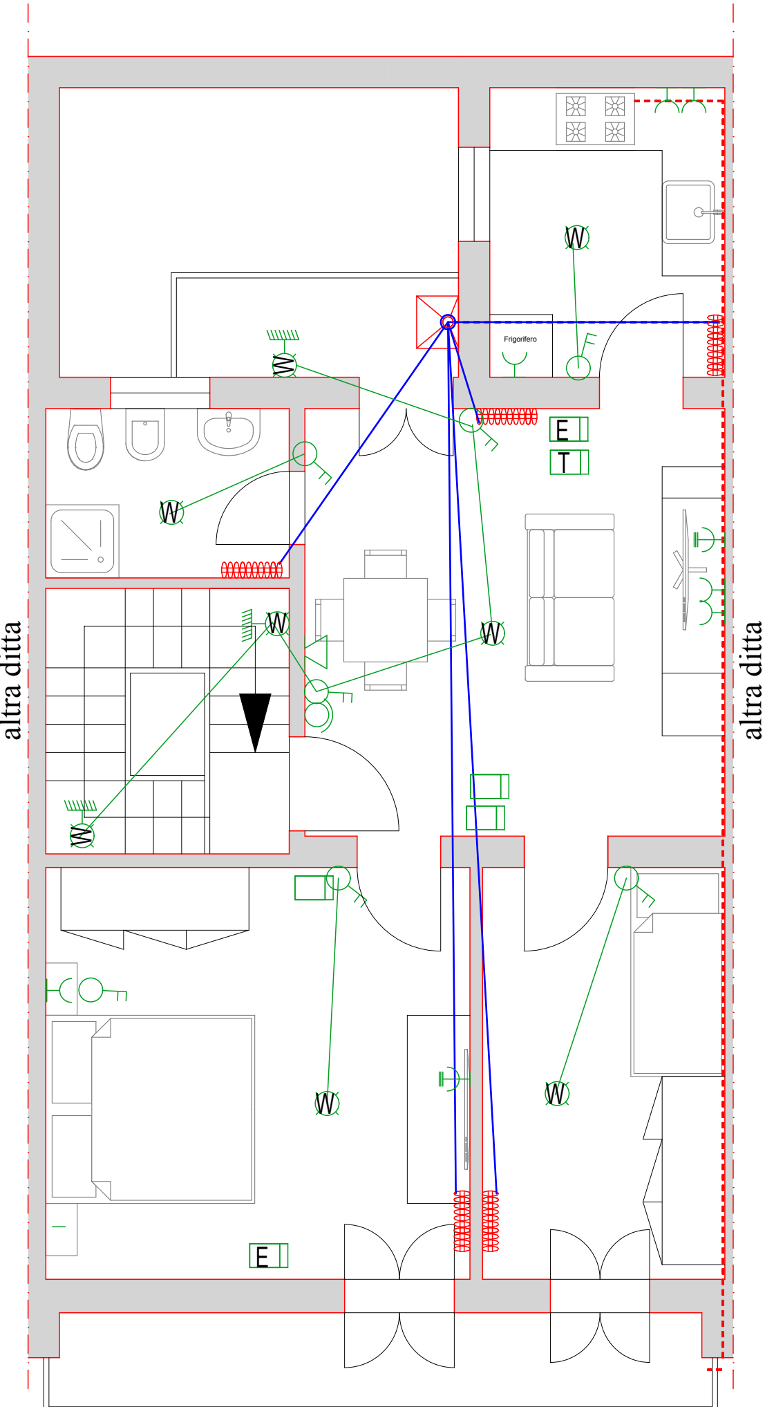
Impianti metano al Secondo Piano
