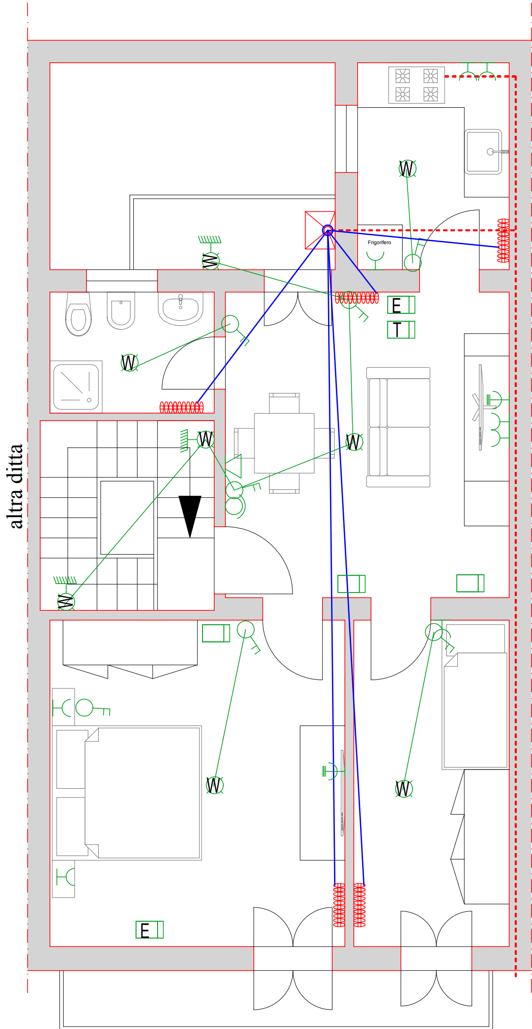
Impianto metano al Primo Piano
