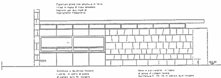
PROSPETTO A-B 1:50
