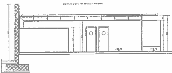
SEZIONE E-E 1:50
