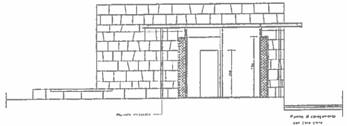
SEZIONE E-D 1:50
