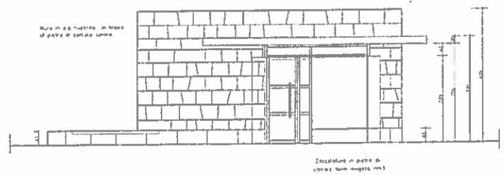
PROSPETTO G-B 1:50
