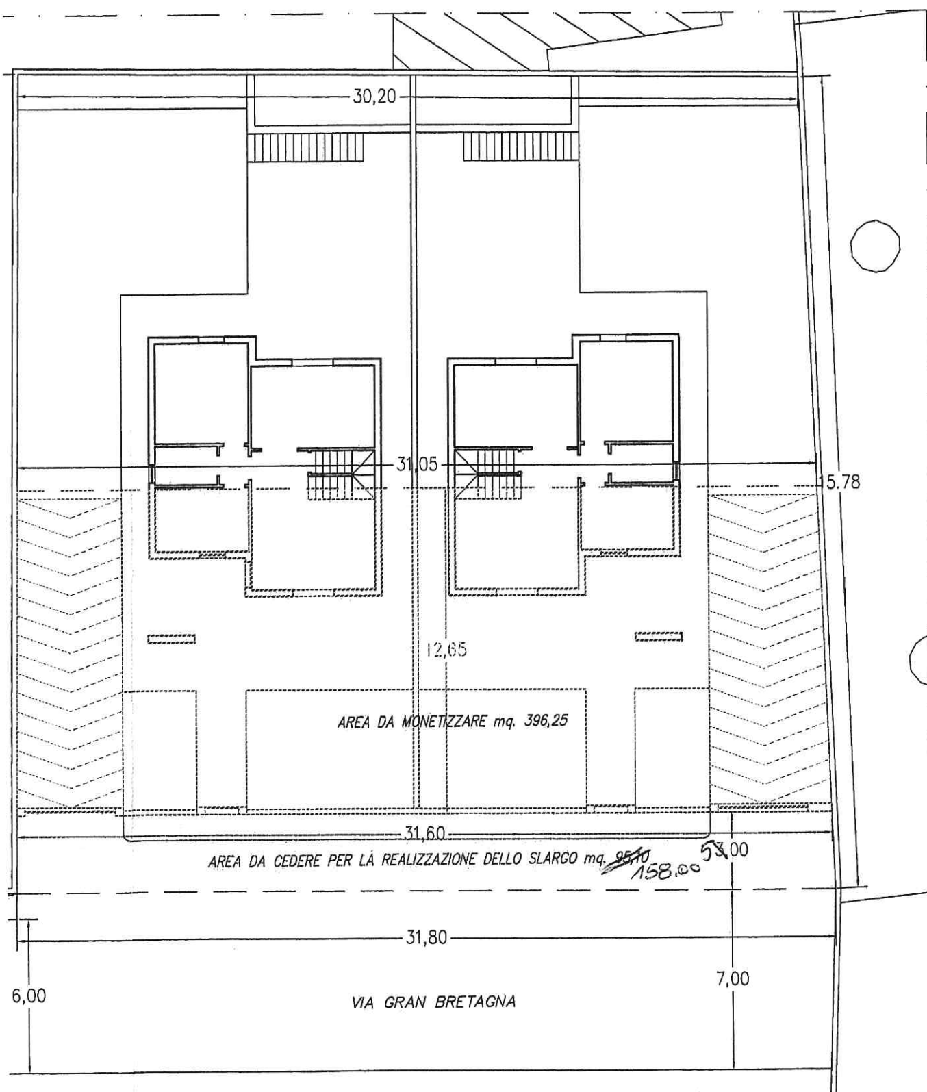
PLANIMETRIA DEL LOTTO scala 1:200
