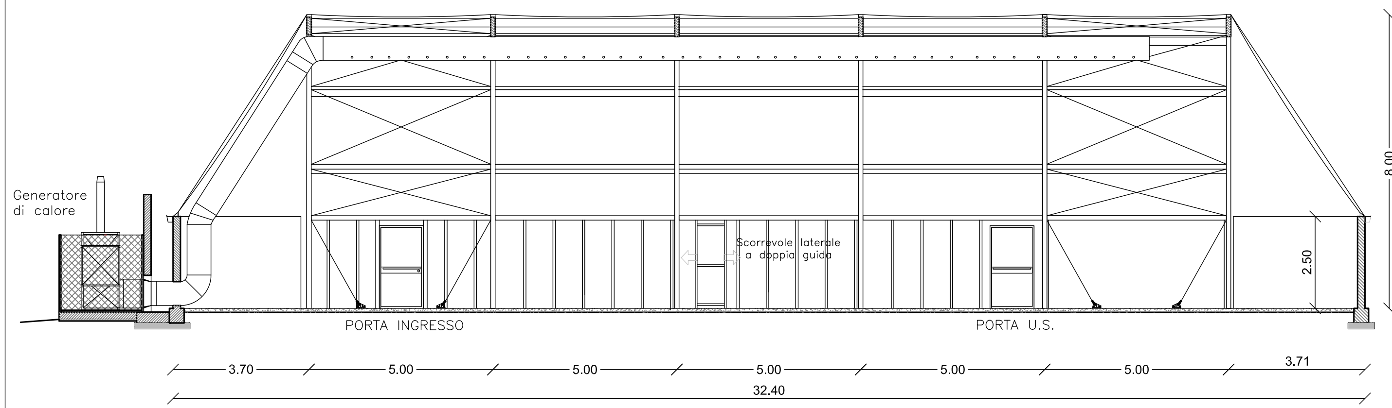
Sezione A-A
