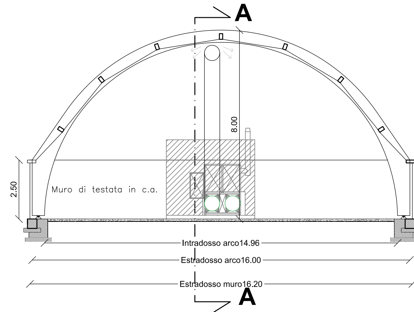
Sezione B-B
