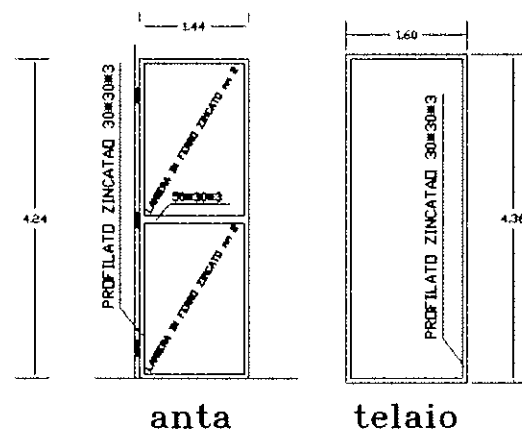
PARTICOLARE PORTA IN FERRO ZINCATO
