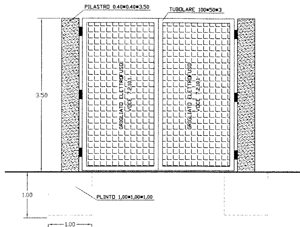
PARTICOLARE CANCELLO IN FERRO ZINCATO
