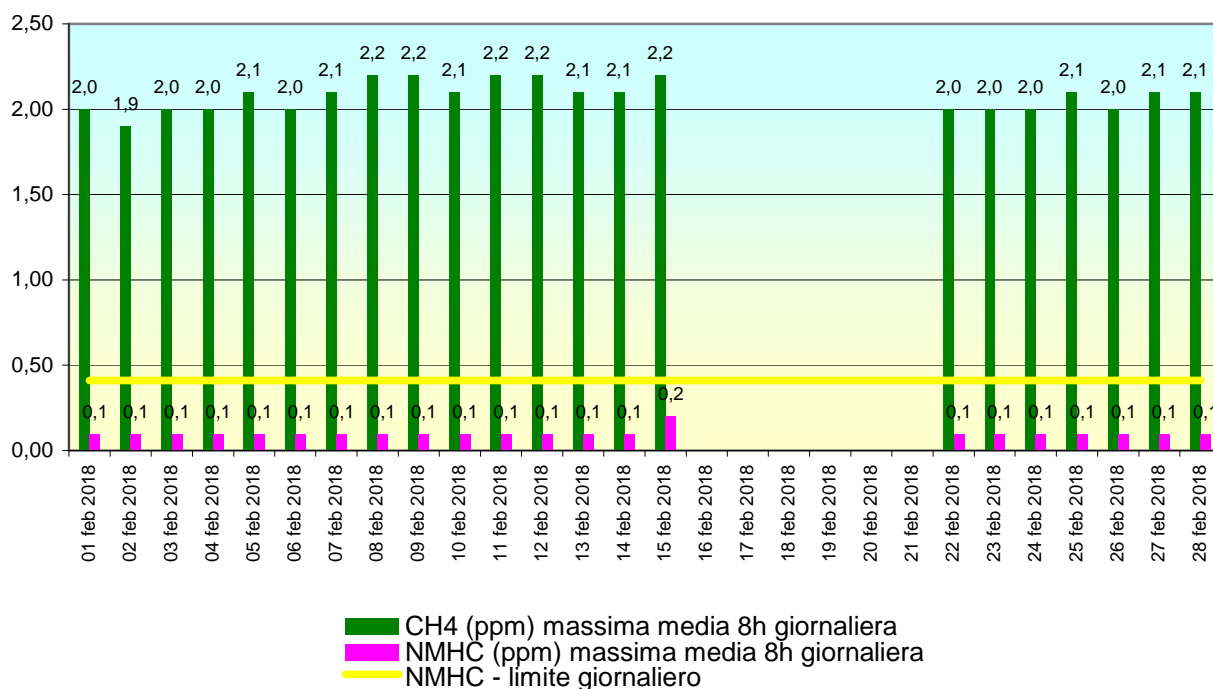
Stazione RG05 MARINA DI RAGUSA, periodo: 01 feb 2018-28 feb 2018 - Dati validati
