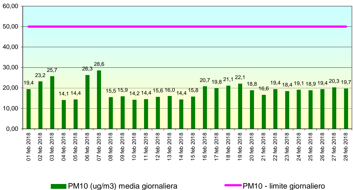
Stazione RG05 MARINA DI RAGUSA, periodo: 01 feb 2018-28 feb 2018 - Dati validati
