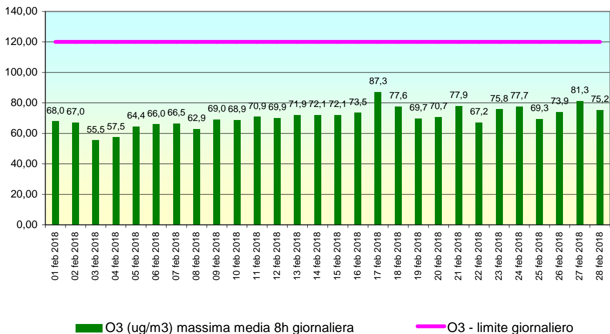
Stazione RG01 CAMPO ATLETICA, periodo: 01 feb 2018-28 feb 2018 - Dati validati
