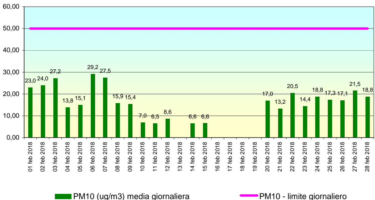
Stazione RG03 VILLA ARCHIMEDE, periodo: 01 feb 2018-28 feb 2018 - Dati validati
