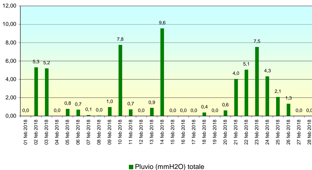
Stazione RG03 VILLA ARCHIMEDE, periodo: 01 feb 2018-28 feb 2018 - Dati validati
