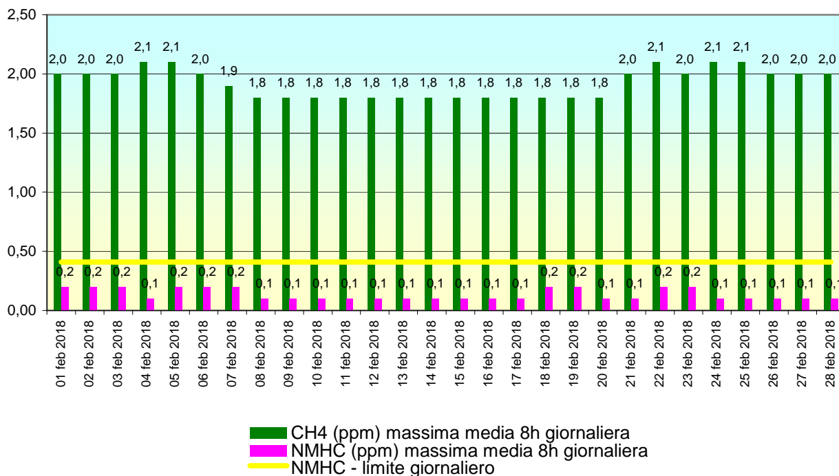
Stazione RG01 CAMPO ATLETICA, periodo: 01 feb 2018-28 feb 2018 - Dati validati
