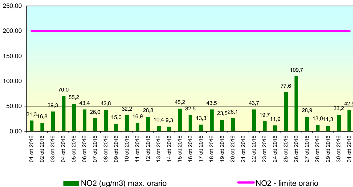
Stazione RG03 VILLA ARCHIMEDE, periodo: 01 ott 2016-31 ott 2016 - Dati validati
