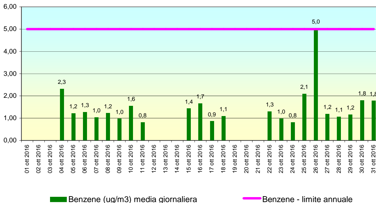
Stazione RG03 VILLA ARCHIMEDE, periodo: 01 ott 2016-31 ott 2016 - Dati validati
