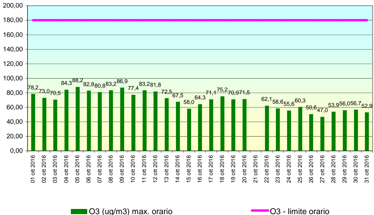
Stazione RG03 VILLA ARCHIMEDE, periodo: 01 ott 2016-31 ott 2016 - Dati validati
