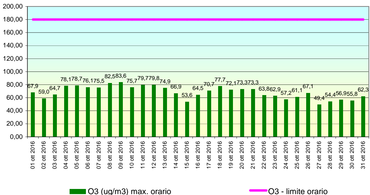
Stazione RG01 CAMPO ATLETICA, periodo: 01 ott 2016-31 ott 2016 - Dati validati
