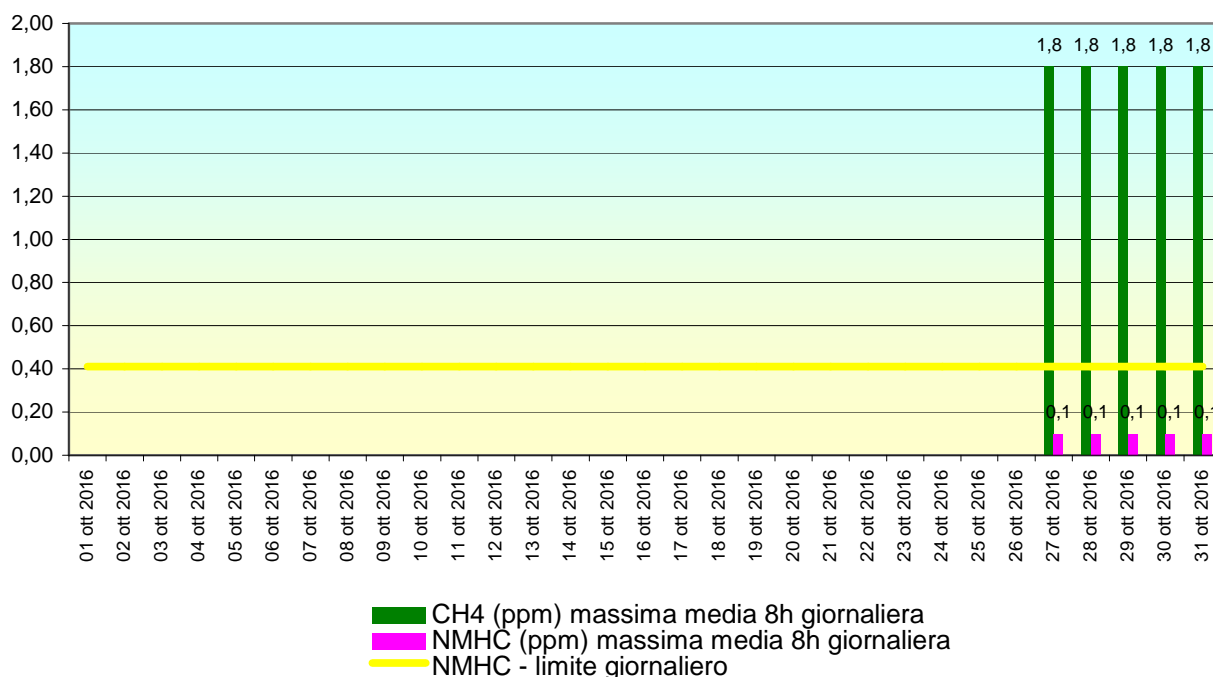
Stazione RG05 MARINA DI RAGUSA, periodo: 03 ott 2016-31 ott 2016 - Dati validati
