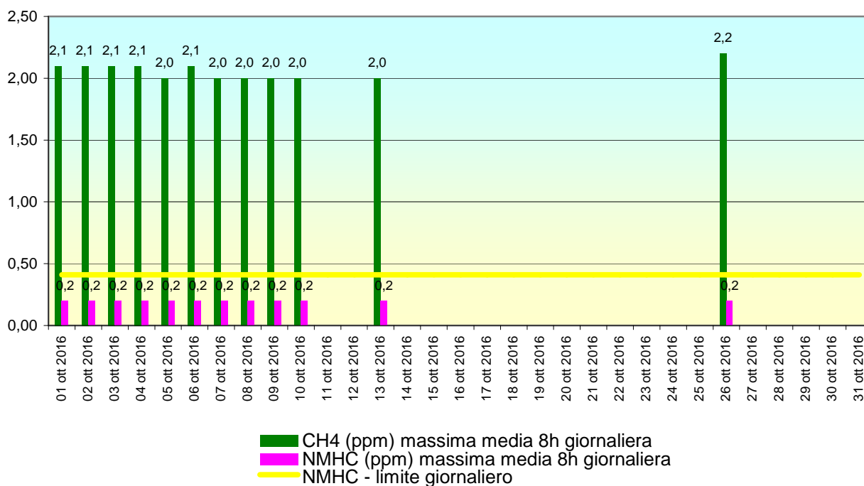
Stazione RG01 CAMPO ATLETICA, periodo: 01 ott 2016-31 ott 2016 - Dati validati
