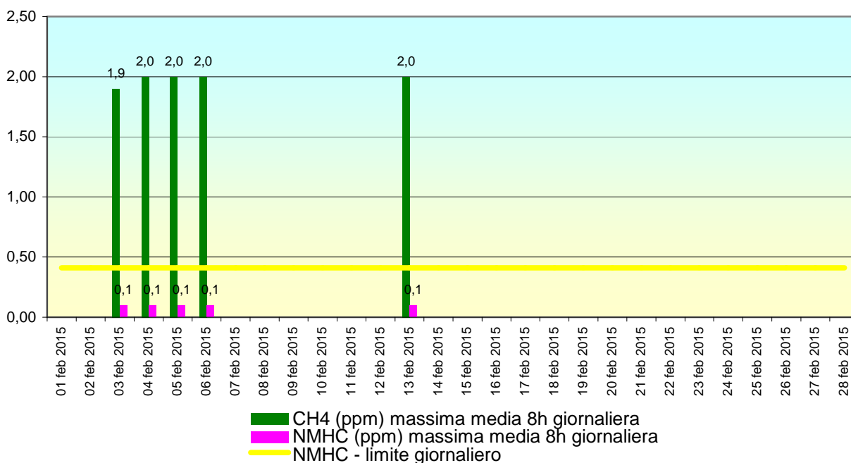
Stazione RG05 MARINA DI RAGUSA, periodo: 01 feb 2015-28 feb 2015 - Dati validati
