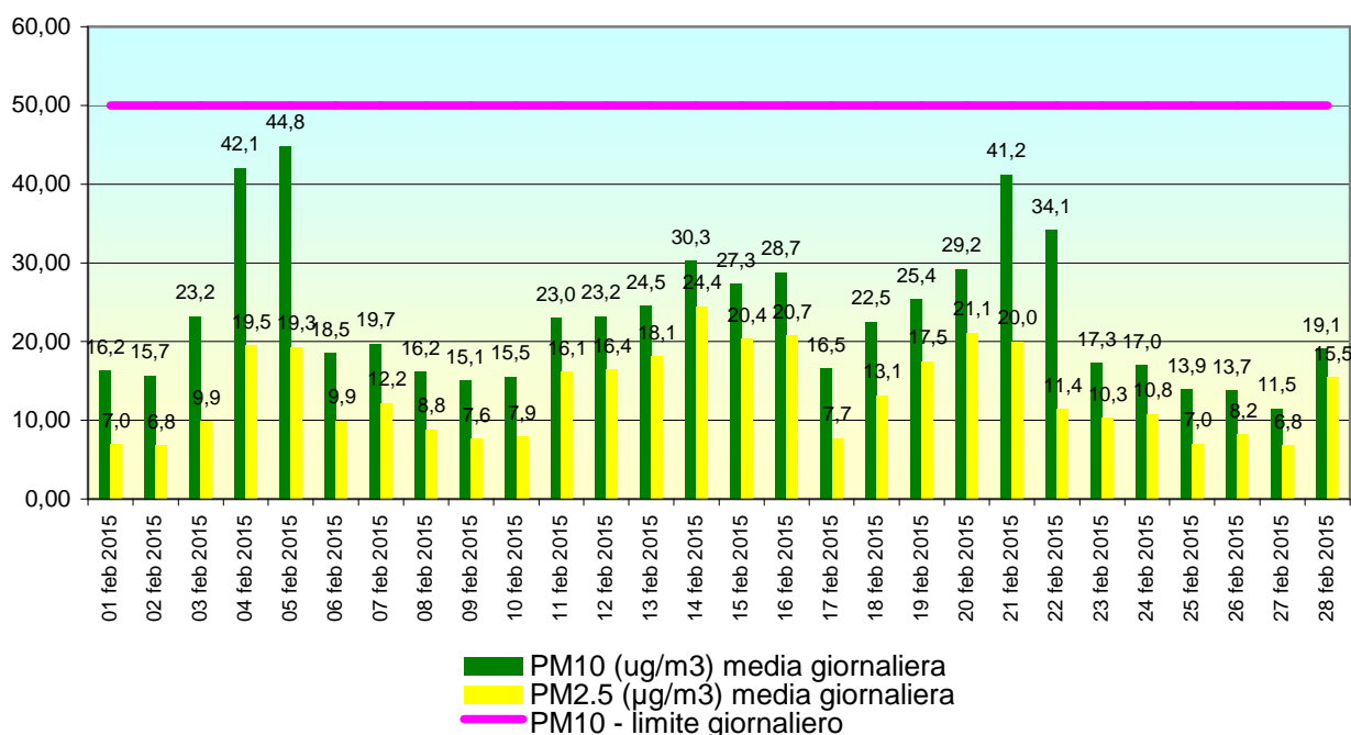
Stazione RG01 CAMPO ATLETICA, periodo: 01 feb 2015-28 feb 2015 - Dati validati
