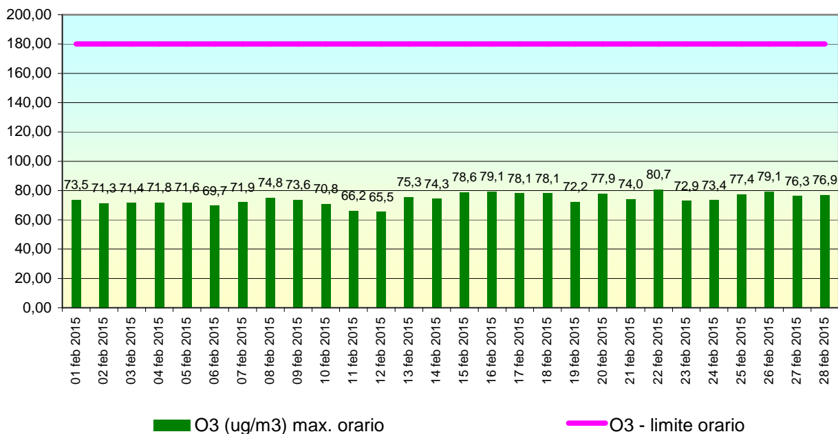
Stazione RG01 CAMPO ATLETICA, periodo: 01 feb 2015-28 feb 2015 - Dati validati
