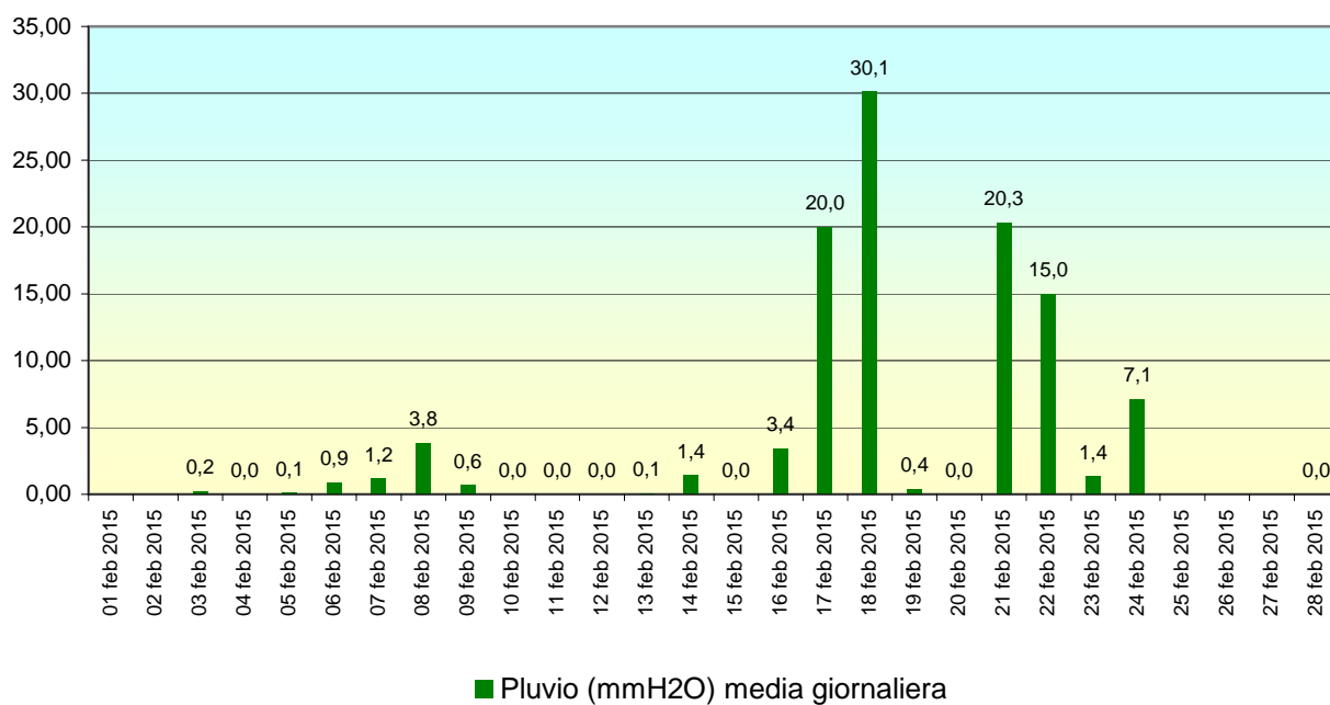
Stazione RG03 VILLA ARCHIMEDE, periodo: 01 feb 2015-28 feb 2015 - Dati validati
