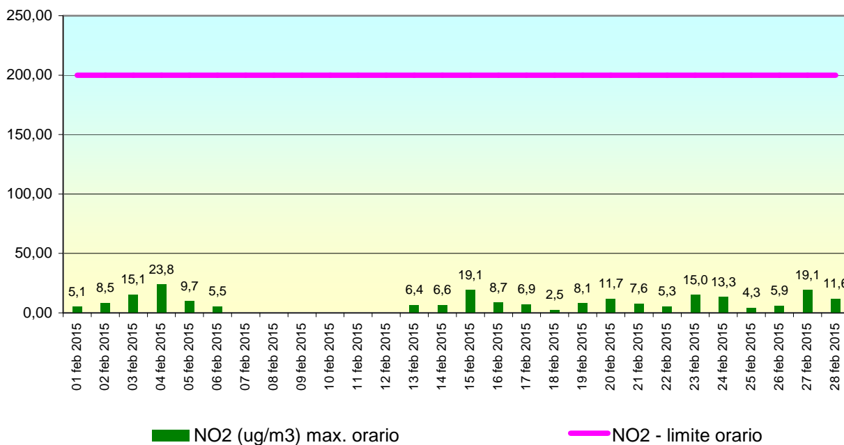
Stazione RG05 MARINA DI RAGUSA, periodo: 01 feb 2015-28 feb 2015 - Dati validati
