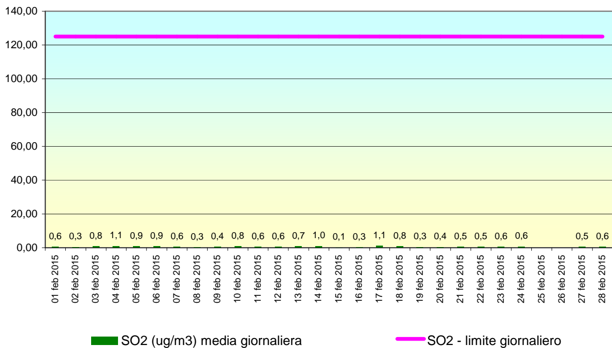
Stazione RG03 VILLA ARCHIMEDE, periodo: 01 feb 2015-28 feb 2015 - Dati validati
