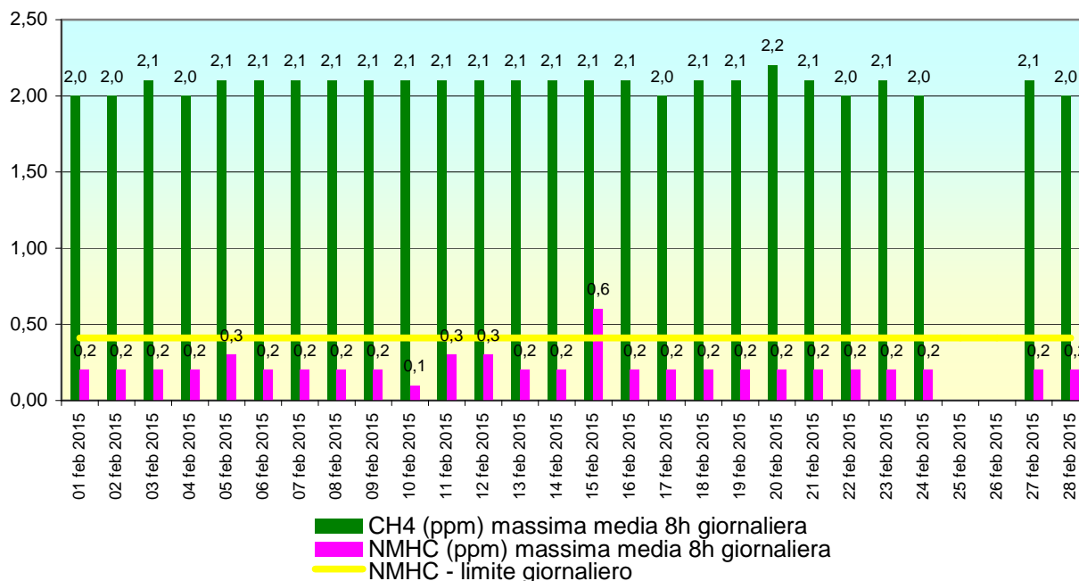
Stazione RG03 VILLA ARCHIMEDE, periodo: 01 feb 2015-28 feb 2015 - Dati validati
